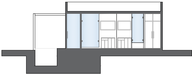
SECCIÓN A-A'/SECTIONAL ELEVATION A-A'
